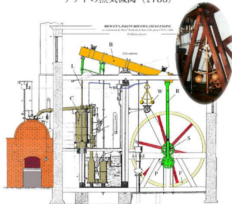
ワットの蒸気機関 (1788)
