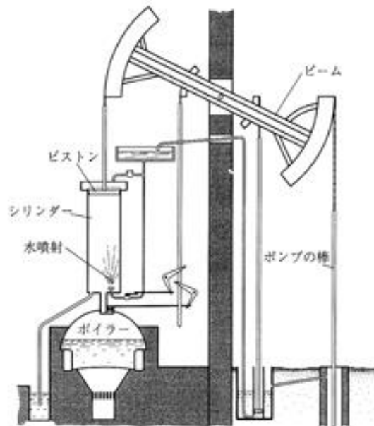
ニューコメンの蒸気機関 (1712年)
